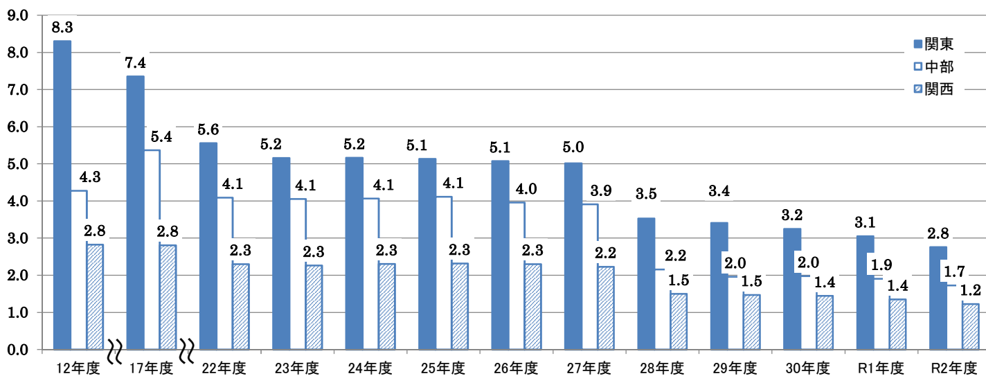
図3 地域別のVOC排出量の推移
