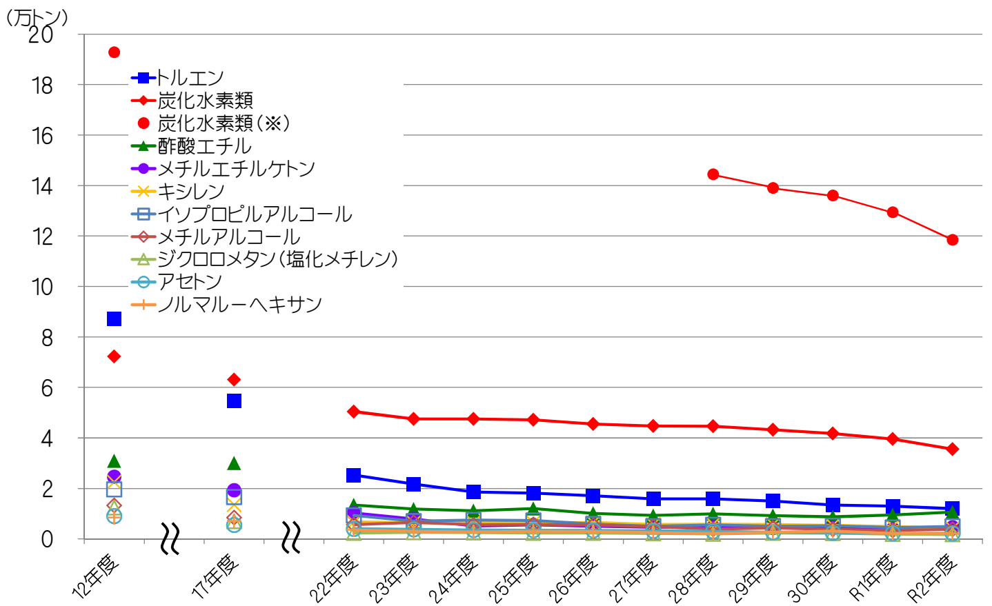
図4 物質別のVOC排出量の推移
