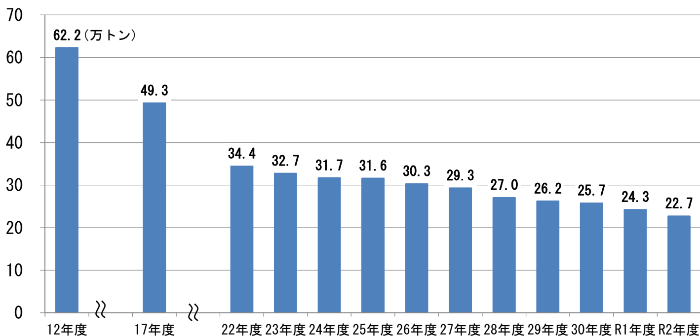
図1 自主的取組における全国のVOC排出量の推移
