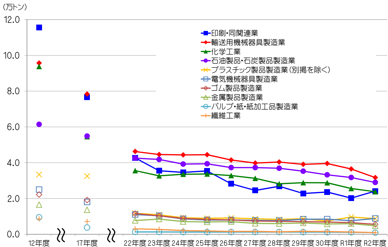
図2 業種別のVOC排出量の推移
